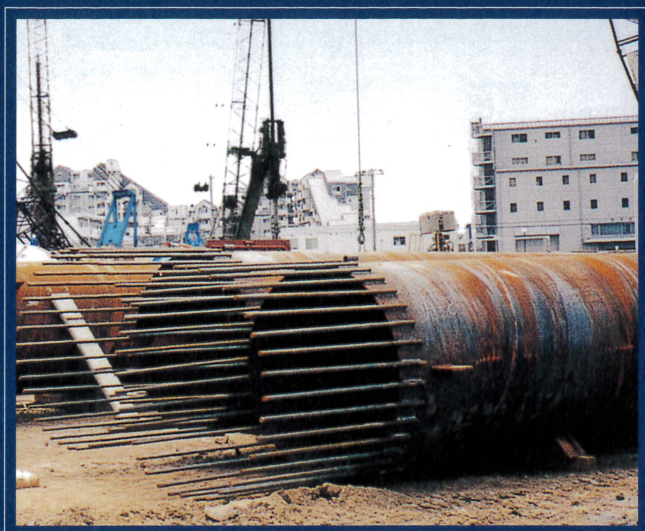
■SB耐震杭 杭頭接合部
